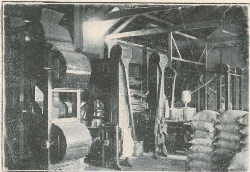
Aspecto interno do mesmo predio, vendo-se os importantes machinarios para o beneficiamento do café.
